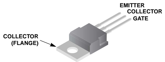
JEDEC TO-220AB
