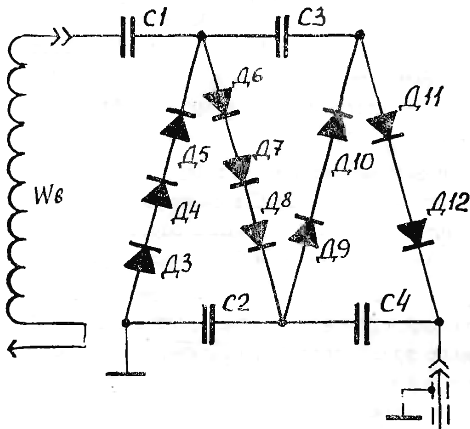
Рис. 7. Схема электрическая принципиальная выпрямителя напряжения
