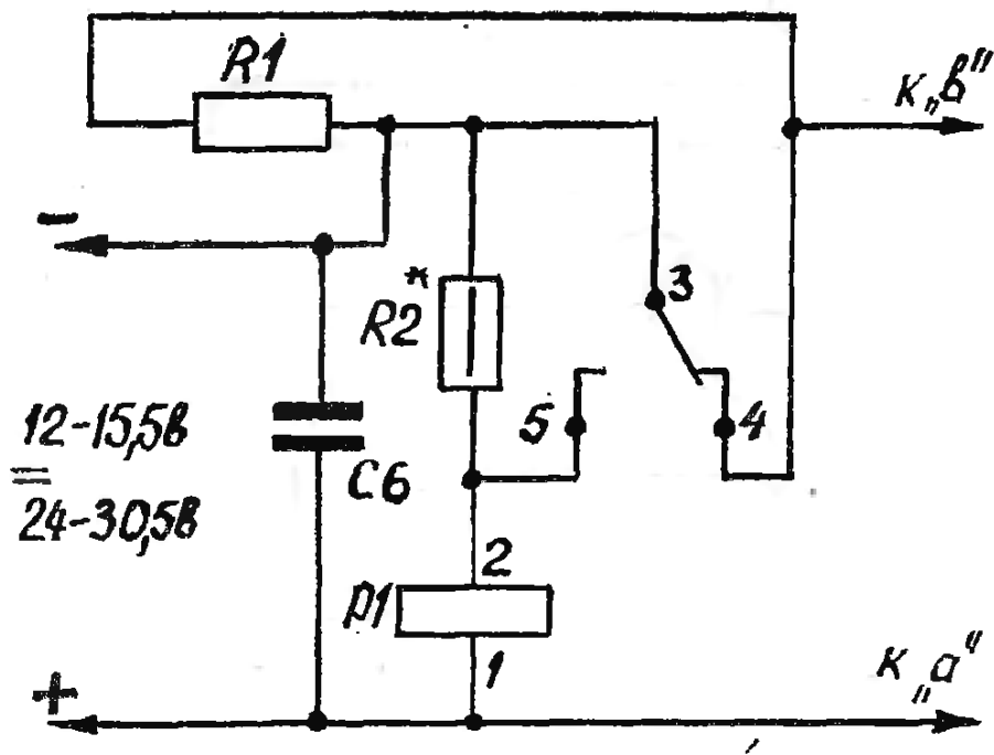
Рис. 4. Схема принципиальная электрическая ограничителя напряжения
