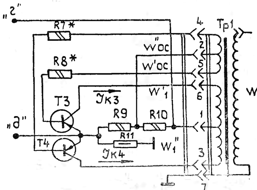
Рис. 6. Схема электрическая принципиальная преобразователя напряжения
