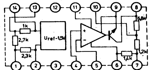
Schemat wewnętrzny
