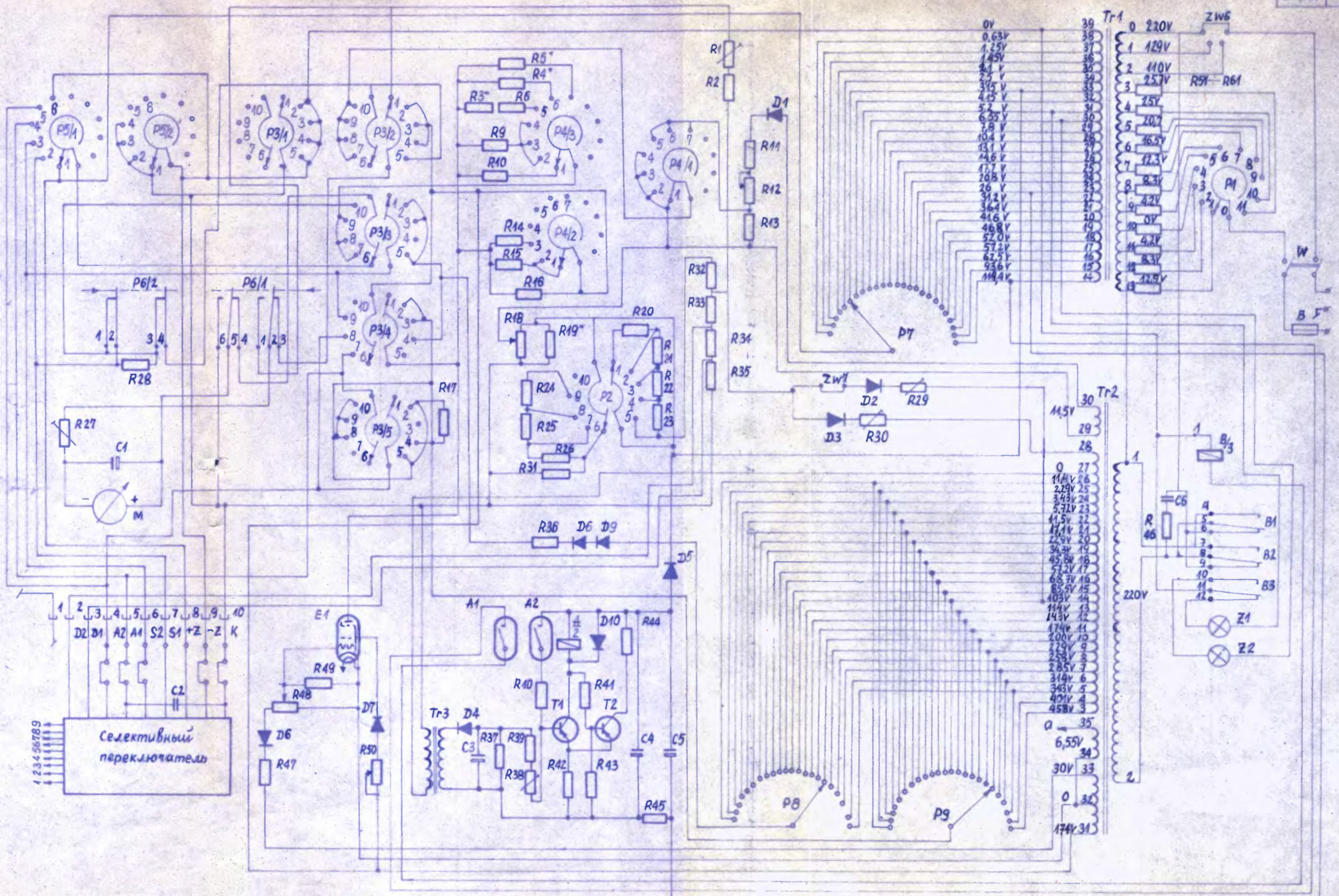
Измеритель электронных ламп ИЭД-Т-508. Электрическая схема
