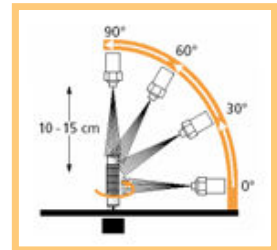
IP69K teszt
