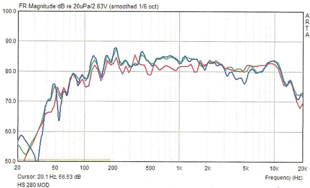
A mérsek 1méter magasan és 0,65méter távolságra elhelyezett mikrofonnal az előlap közepére irányítva történt, miközben a magasság le és föl 10cm renként változott.
