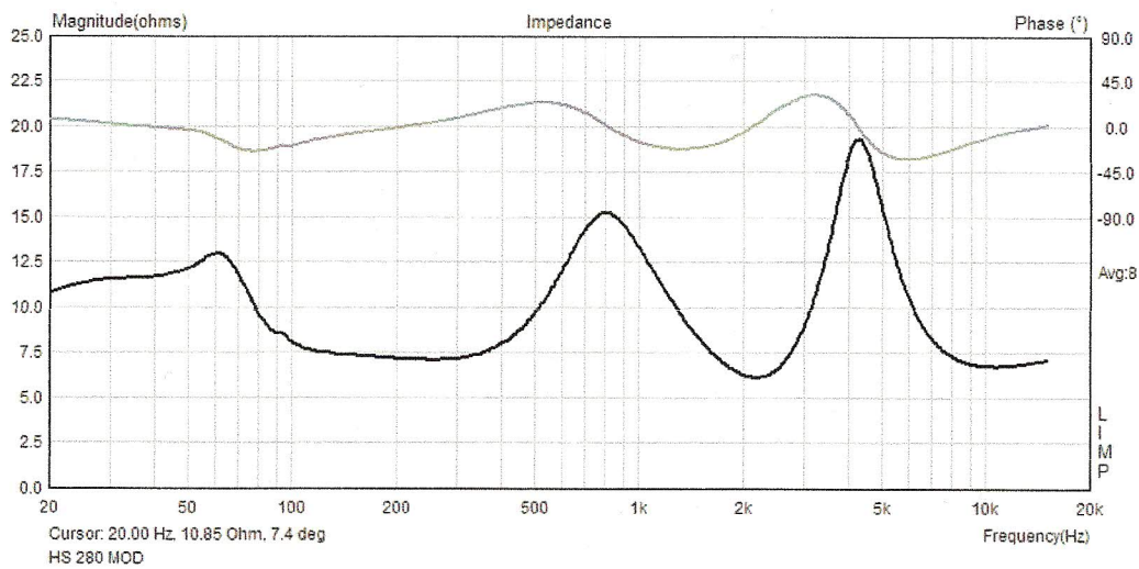
A módosított szűrőváltó impedancia és fázismenete.
