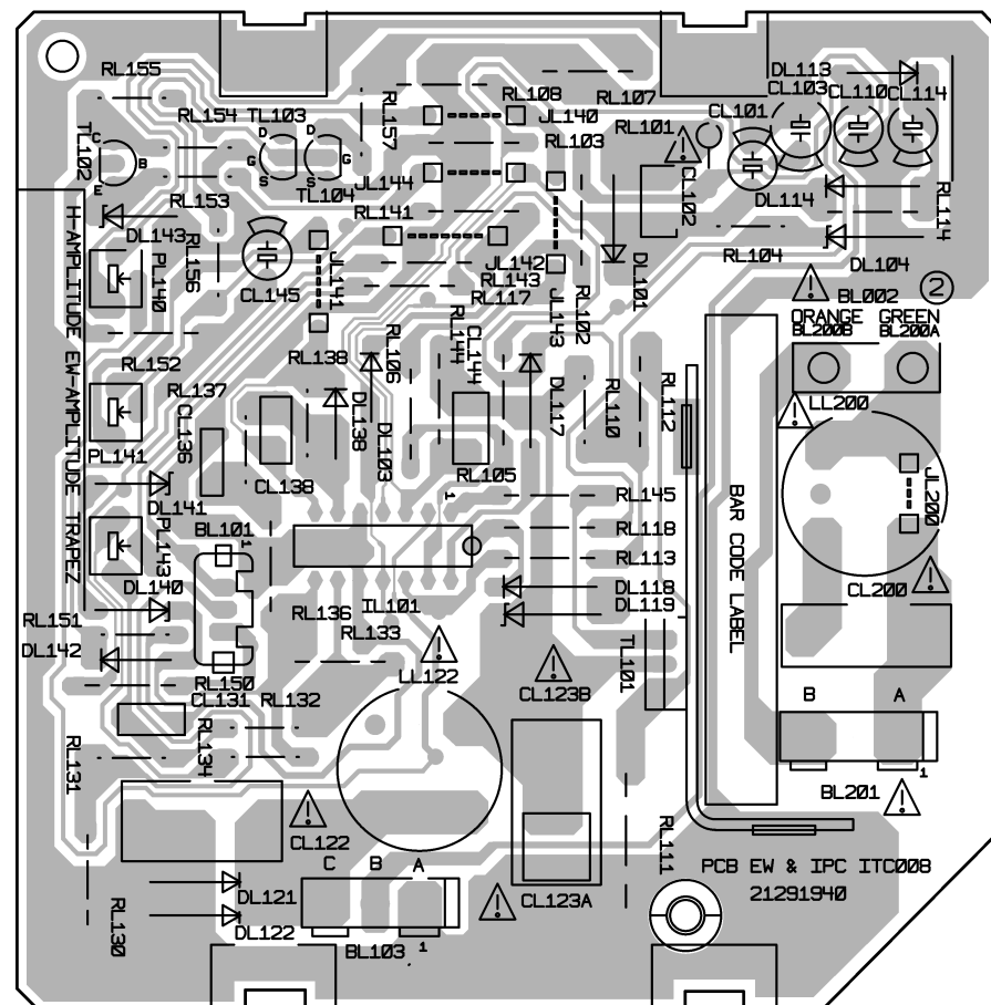
COMPONENT SIDE - CÔTE COMPOSANTS - BESTÜCKUNGSSEITE - LATO COMPONENTI - LADO COMPONENTES
