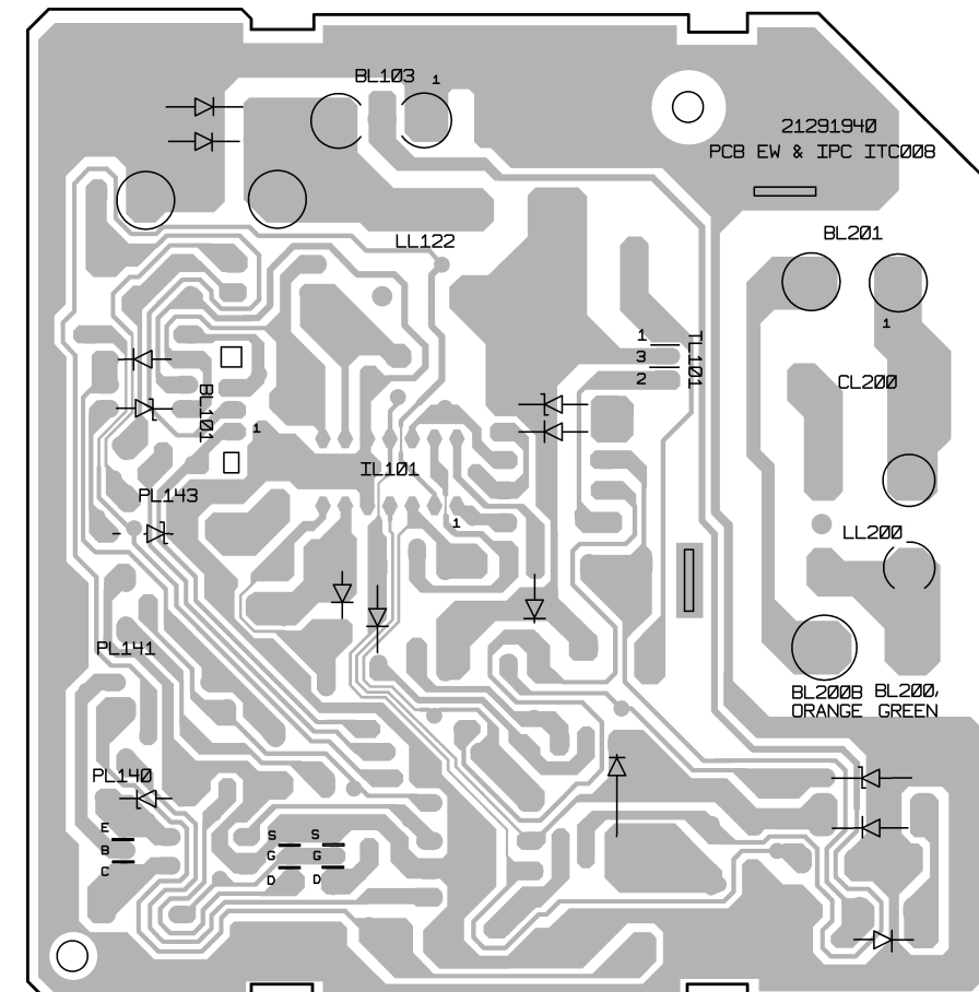
SOLDER SIDE - CÔTE SOUDURES - LÖTSEITE - LATO SALDATURE - LADO SOLDADURAS
