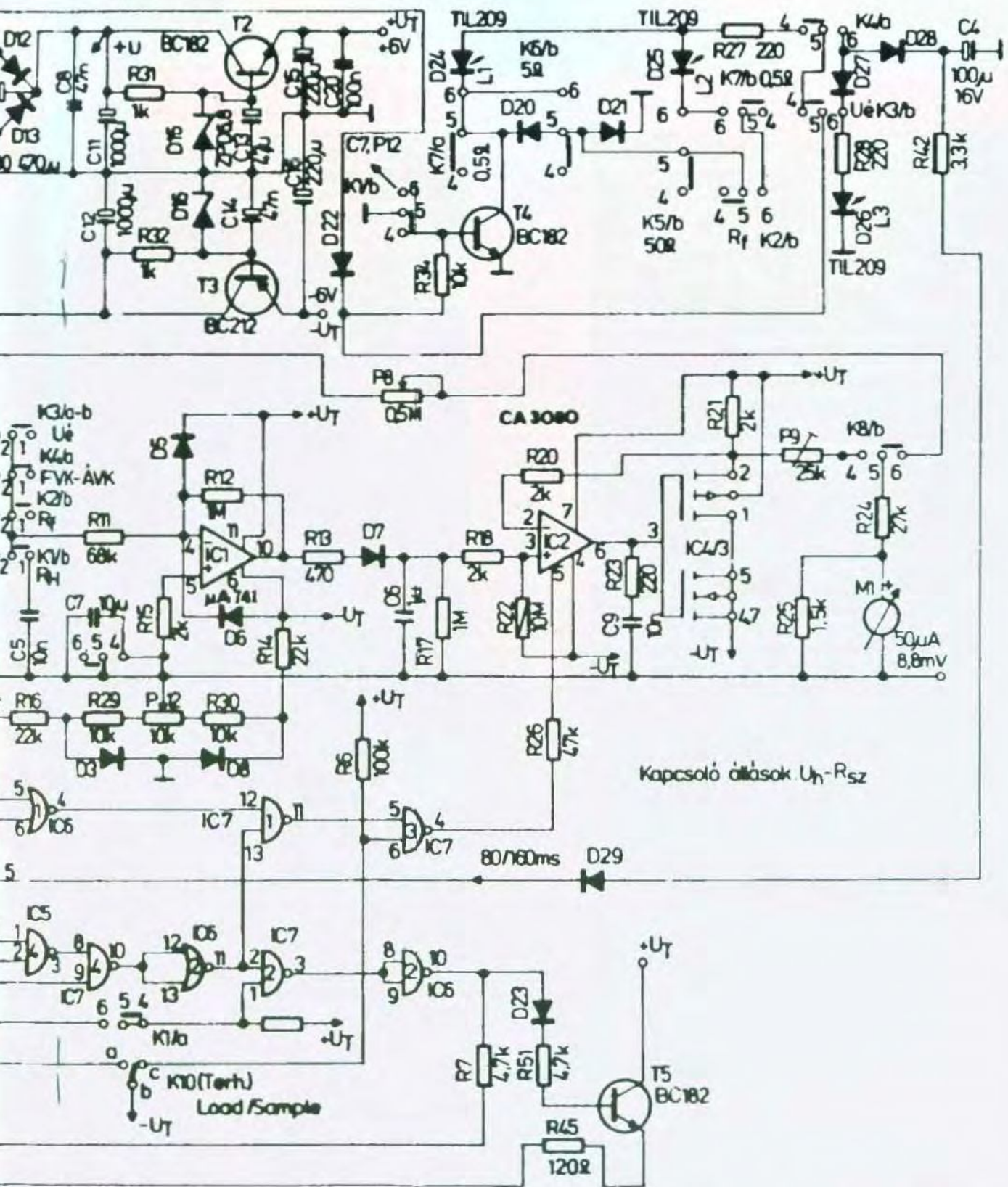
SAL hordozható érintésvédelmi mérő- és ellenőrző műszer
