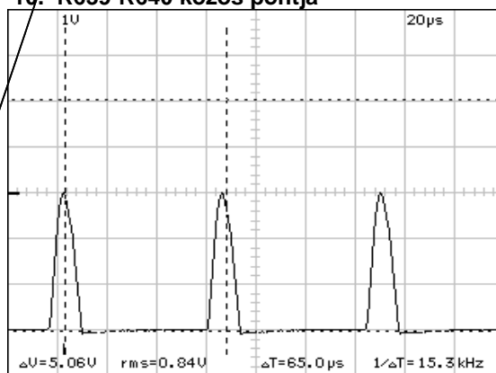
10. R639-R640 közös pontja
