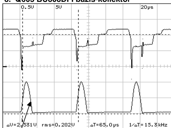
8. Q603 BU808DFI bázis-kollektor
