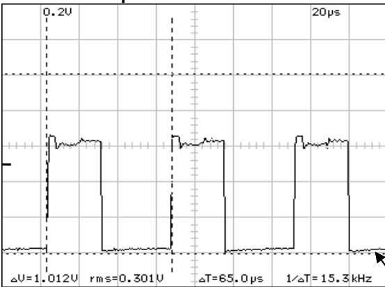
1. STV2248C pin 40. Hout
