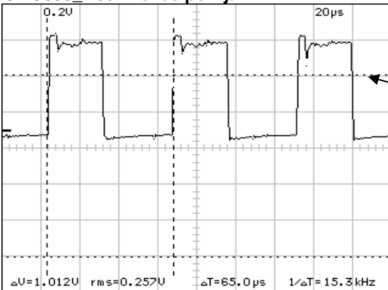
3. C635 R662 közös pontja
