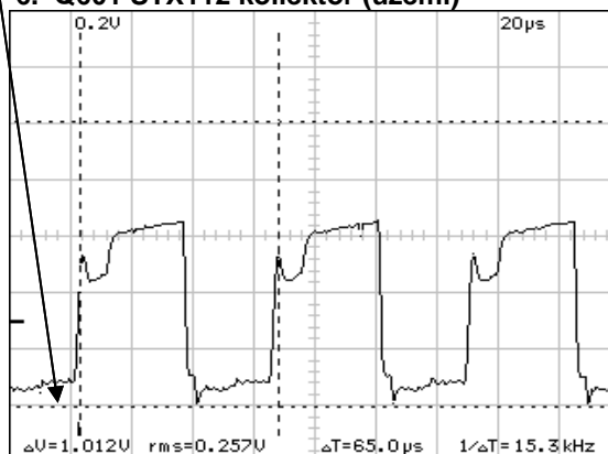
6. Q601 STX112 kollektor (üzemi)
