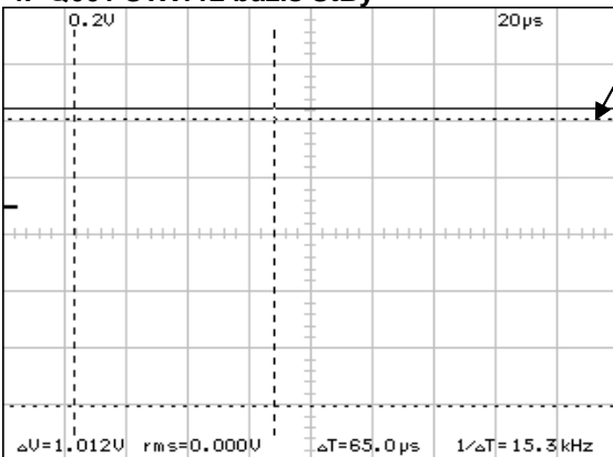
4. Q601 STX112 bázis StBy
