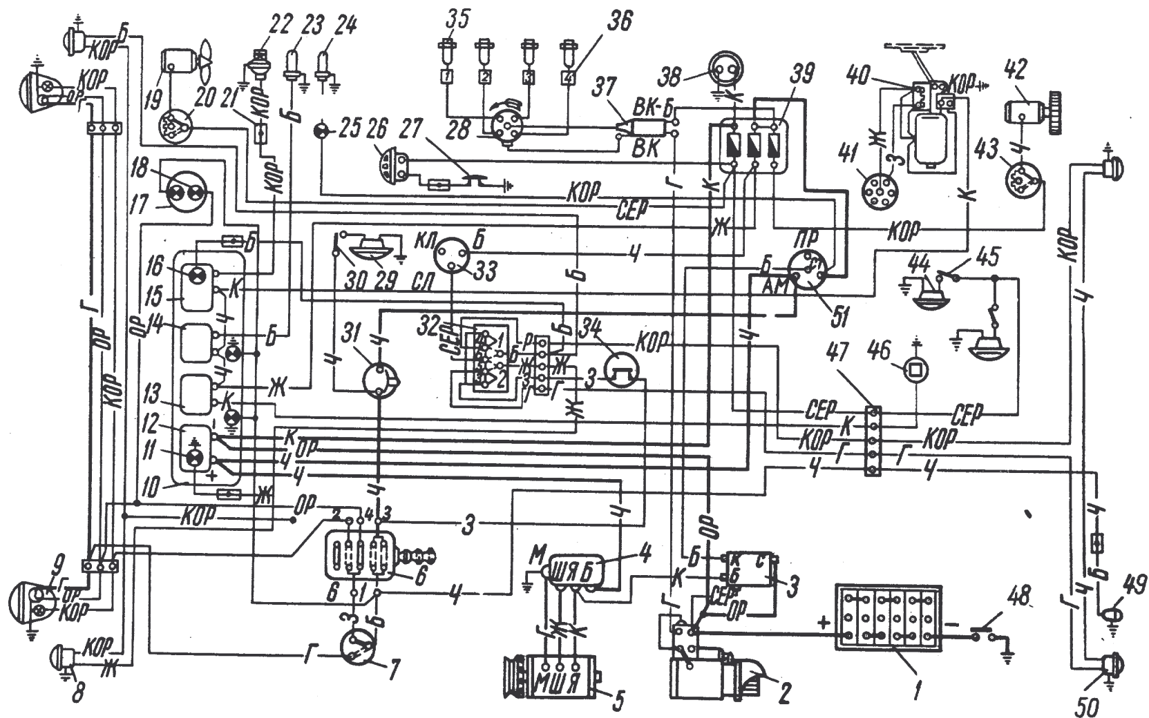
52. ábra. Az UAZ-452 és UAZ-452V gépkocsi villamos berendezésének kapcsolási rajza.
