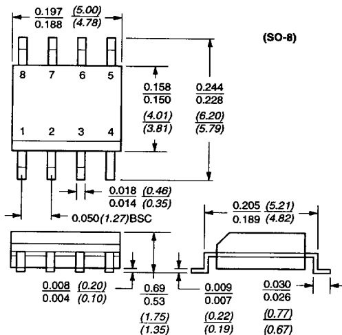
SO-8
