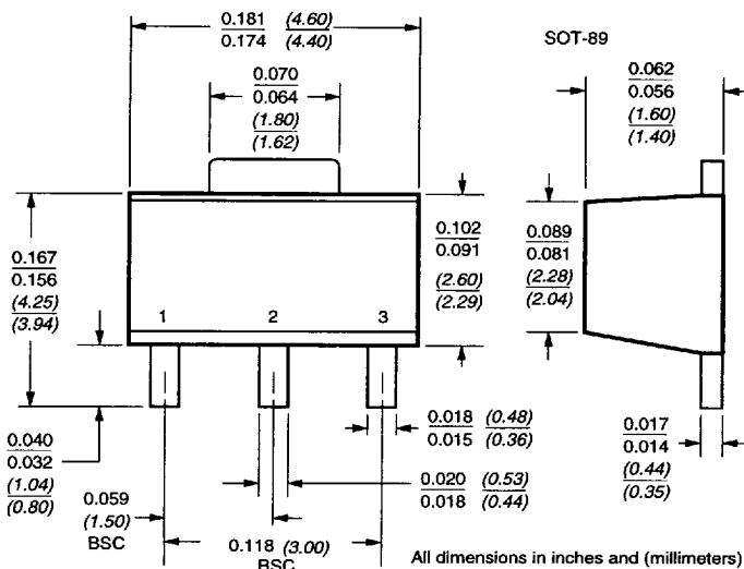
SOT-89
