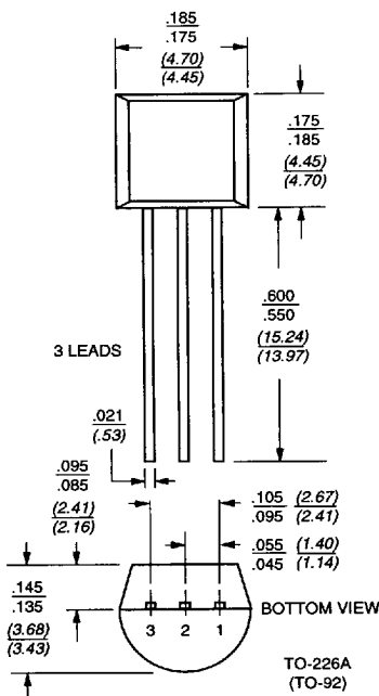
TO-92 (TO-226A)
