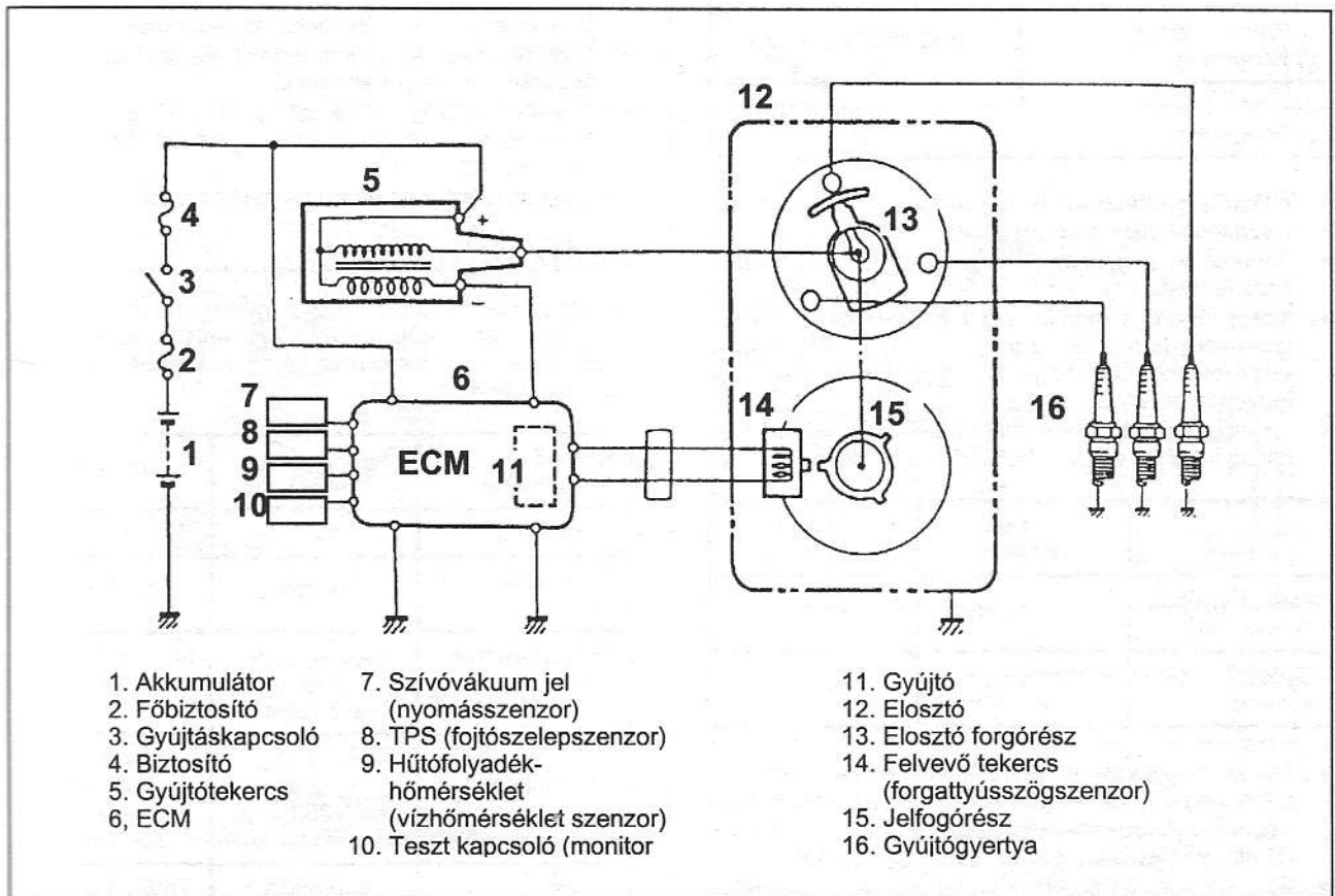
11-1 ábra Az elektronikus vezérlésű gyújtás (ESA) kapcsolási rajza
