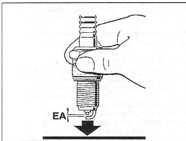
11-2 ábra A gyújtógyertya elektródahézagja
